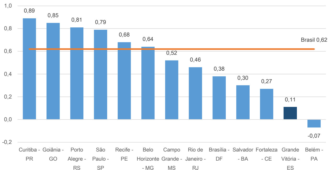
Gráfico 1 – Variação (%) mensal - Brasil, regiões metropolitanas e municípios IPCA - Julho de 2015
