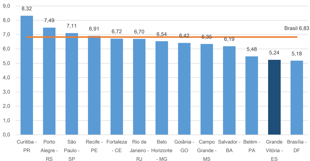
Gráfico 3 – Variação (%) acumulada no ano - Brasil, regiões metropolitanas e municípios IPCA - Julho de 2015
