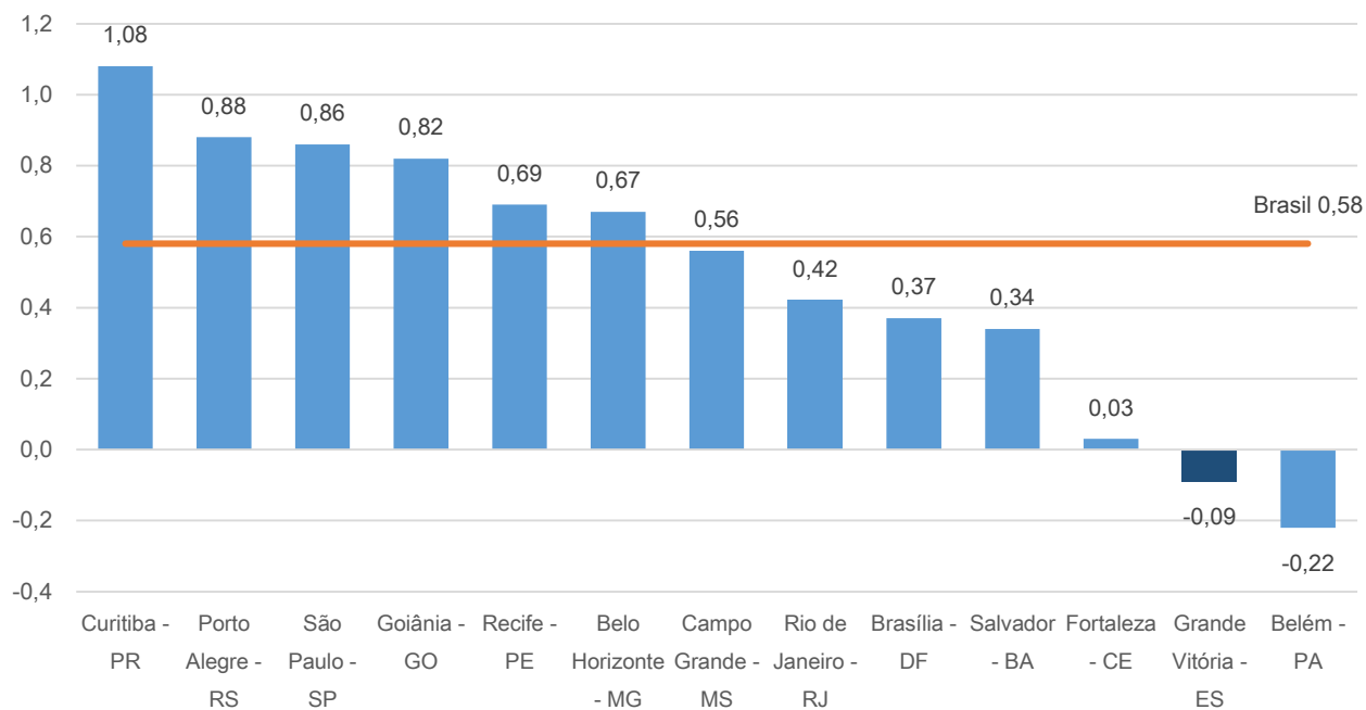
Gráfico 4 – Variação (%) mensal - Brasil, regiões metropolitanas e municípios INPC - Julho de 2015
