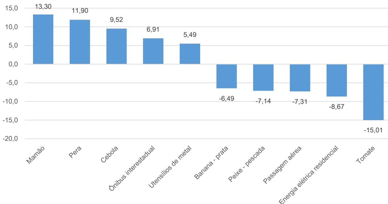
Gráfico 2 – Produtos e serviços com as maiores variações (%) de preço na Grande Vitória IPCA – Julho de 2015
