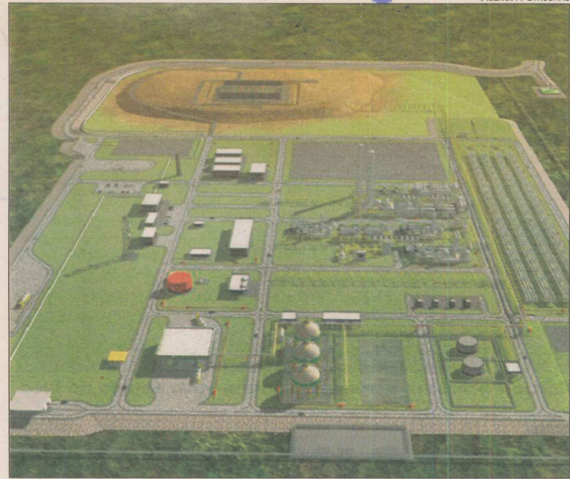
Projeção gráfica de uma Unidade de Tratamento de Gás
