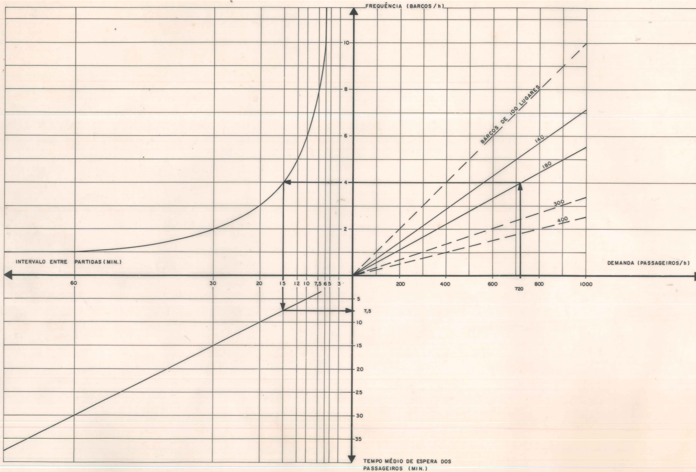
FIGURA 4 : NOMOGRAMA PARA A DETERMINAÇÃO DA CAPACIDADE ÓTIMA DOS BARÇOS.
